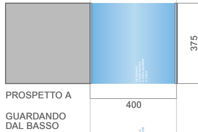
PROSPETTO A stato di progetto
