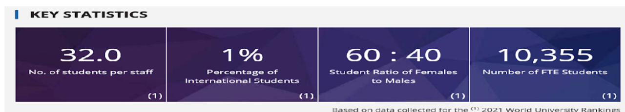
Fig. 3 Elementi dimensionali dell'Università di Foggia rilevati da THE
