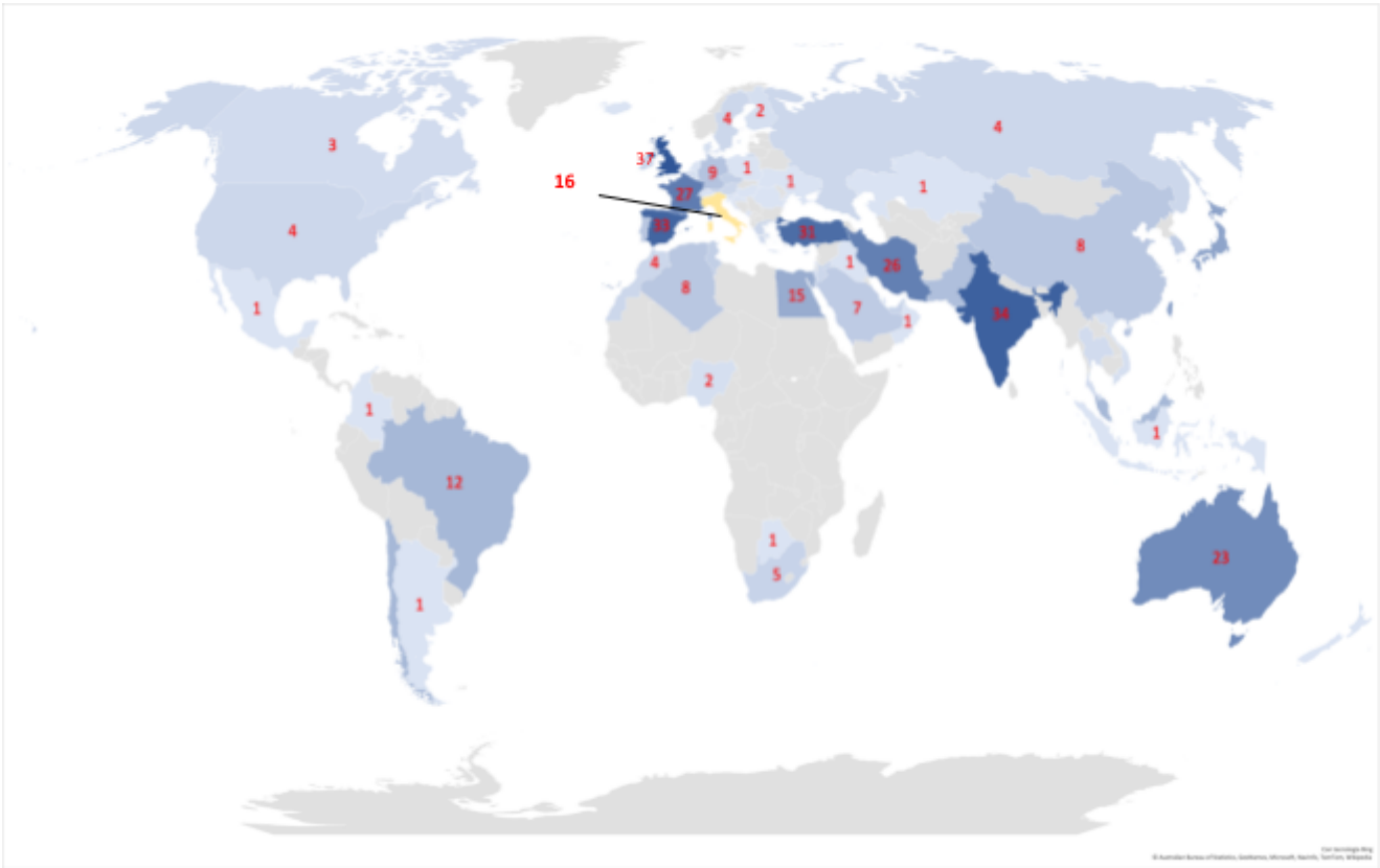
Fig. 2 La classifica Young per rappresentatività geografica delle università partecipanti al ranking
