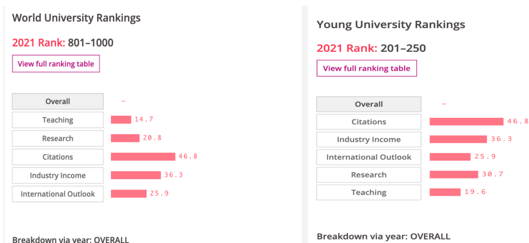
Fig. 4 Posizionamento dell'Università di Foggia con indicatori di valutazione rispetto alle due classifiche di Ranking di THE World e Young.
